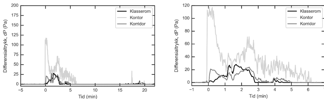
Figur 4-48: Trykkdifferansen mellom hvert av rommene og omgivelsestrykk utenfor bygget for test 10. Venstre figuren viser hele testforløpet. Høyre figuren viser perioden med høyest trykkøkningene.
