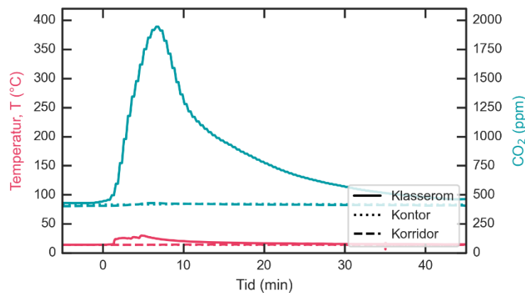
Figur 4-2: Temperatur (rød) og CO 2 konsentrasjon (turkis) i de ulike rommene målt med SD anleggets veggensorer for test 2. Øvre målegrensen for CO 2 var 2000 ppm. Heltrukken linje representerer klasserommet, prikket linje representerer kontoret og stiplet linje representerer korridoren.
