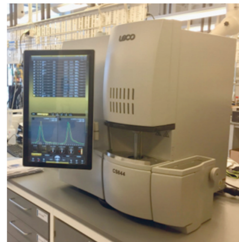
Leco CS844 analyser.
